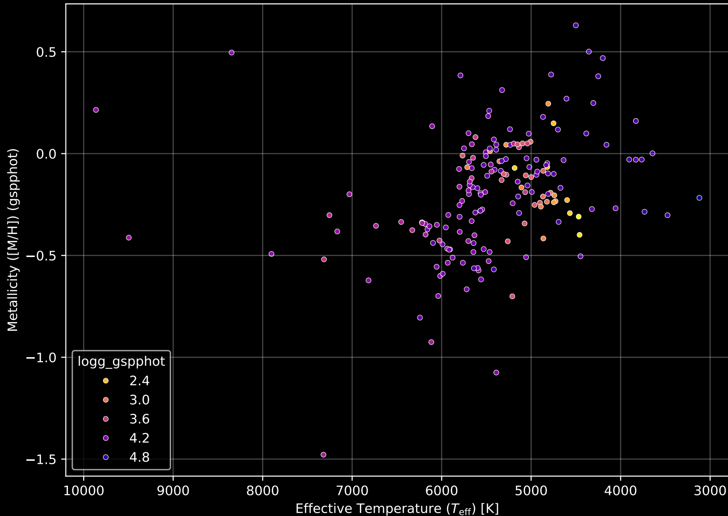
APOGEE DR17 Field: [174+35_MGA] Stellar Population Parameters (n= 184)
